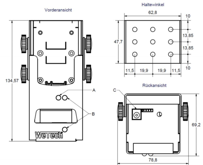
Schemazeichnung WTC692
