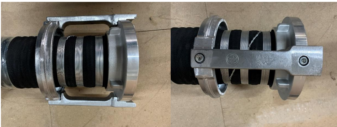
Bild 1: Schnellkupplungsgriffe „Scharfenberg“ am A-Saugschlauch
