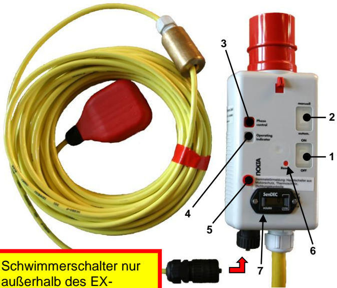
Bild 4: Motorschutzstecker mit Schwimmerschalter
