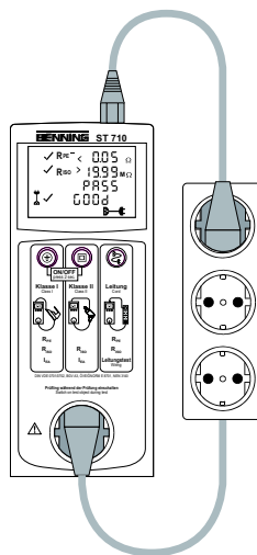
Bild 5b: Prüfung von Leitungen, Mehrfachverteilem und Leitungsroller Fig. 5b: Testing of lines, multiple distributors and cable reels Fig. 5b: Contrôle de câbles, de câbles de distribution multiple et d'enrouleurs de câble Obr. 5b: Zkoušení kabelů, vícenásobných rozvaděčů a kabelových cívek Fig. 5b: Testen van kabels, verdeel dozen en kabelhaspels Rys. 5b: Testowanie kabli, rozdzielnic wielokrotnych i bębnow kablowych
