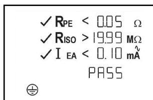
Patrz Rysunek 3: Testy urządzeń klasy ochronnej I (urządzenia z przewodami ochronnymi i dotykającymi się i przewodzącymi częściami, które są podłączone do kabla ochronnego)
