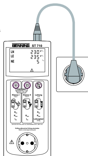
Bild 6: Spannungsmessung an externer Schutzkontaktsteckdose Fig. 6: Voltage measurement on external shock-proof socket Fig. 6: Mesure de tension sur une prise de courant de sécurité externe Obr. 6: Měření napětí na externí zásuvce s ochranným kontaktem Fig. 6: Spanningsmeting aan externe veiligheidswandcontactdoos Rys. 6: Pomiar napięcia na zewnętrznym gniazdku wtykowym z zestykiem ochronnym
