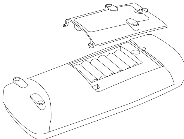
Bild 7: Batteriewechsel Fig. 7: Battery replacement Fig. 7: Remplacement des piles Obr. 7: Výměna baterií Fig. 7: Vervanging van de batterij. Rys. 7: Wymiana baterii
