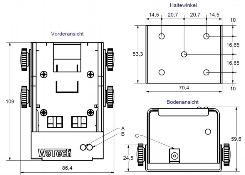
Schemazeichnung WTC620
