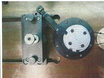
Bild 2: Kupplungsschlüssel – Drehmomentprüfung / Picture 2 Coupling spanner – torque testing
